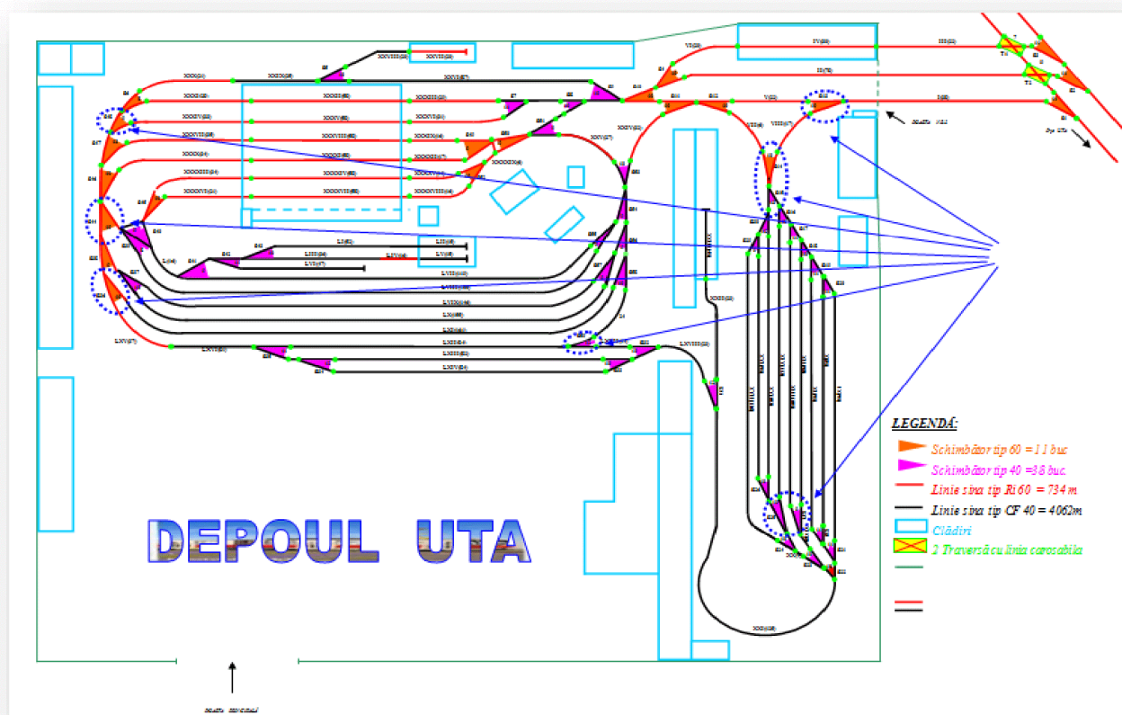
Figura 3.2. Planul general al depoului UTA.
