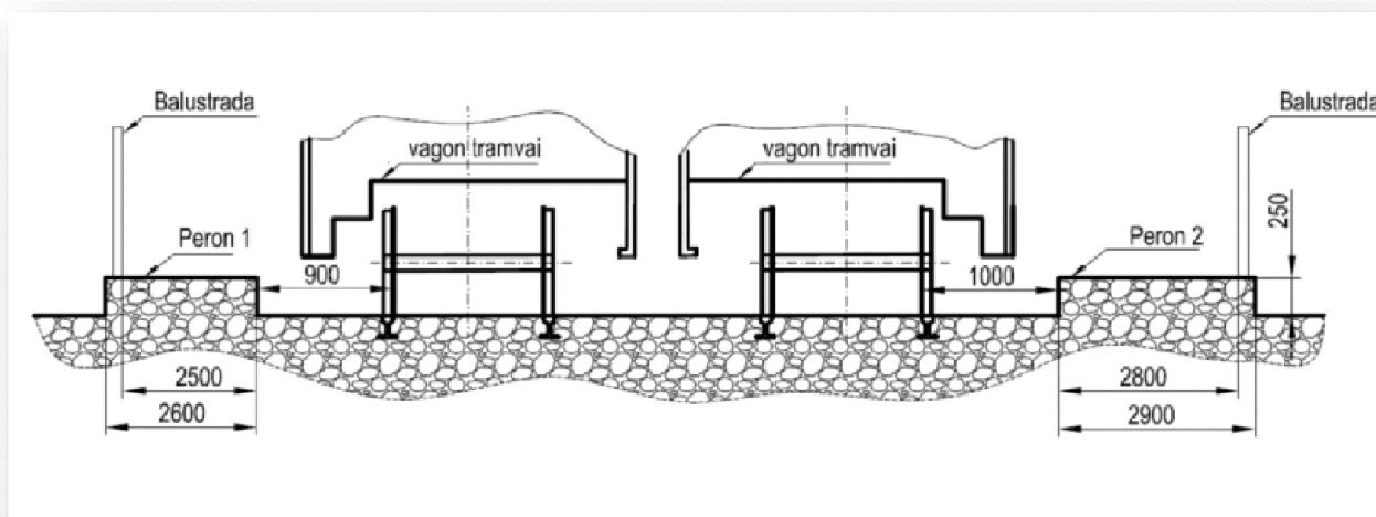
Figura 3.3. Secțiunea transversală în stația Gară.
